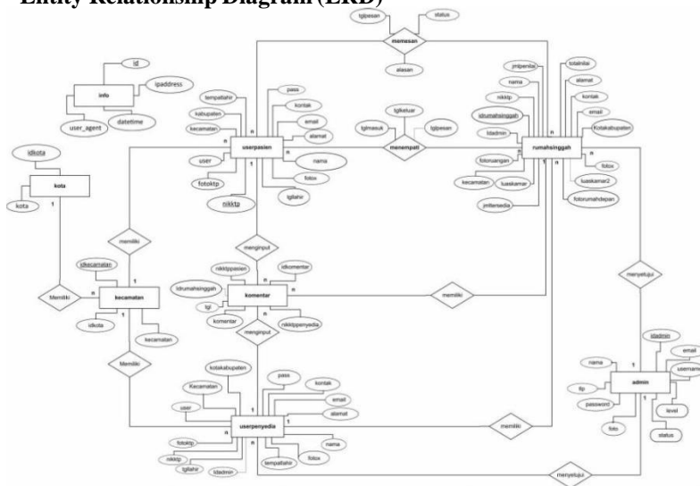
Gambar 6 ERD
