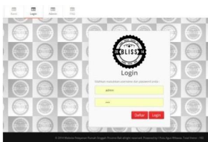
Gambar 6 Halaman Login
