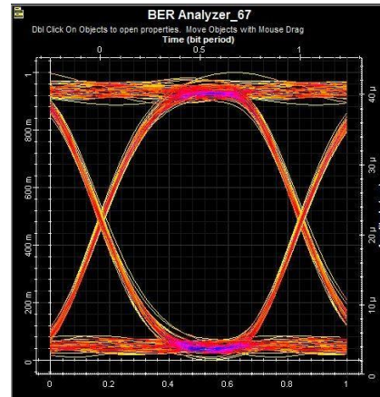
Gambar 4.6 Eye diagram pada modulasi eksternal
