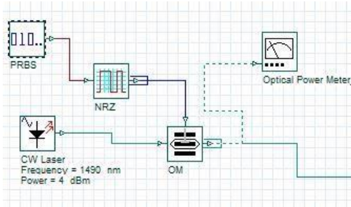
Gambar 3.2 Blok OLT dengan modulasi direct (atas), eksternal (bawah)
