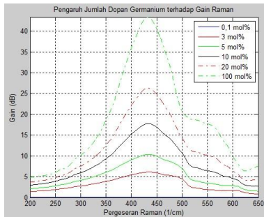
Gambar 4.9 Grafik pengaruh konsentrasi dopant germanium terhadap gain
