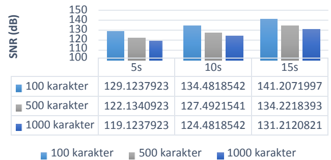
Gambar 4.5 SNR pengujian sistem yang hanya menggunakan pemodelan psychoacoustic
