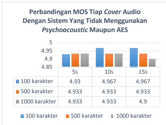
Gambar 4.16 MOS untuk sistem tanpa pemodelan psychoacoustic dan tanpa AES
