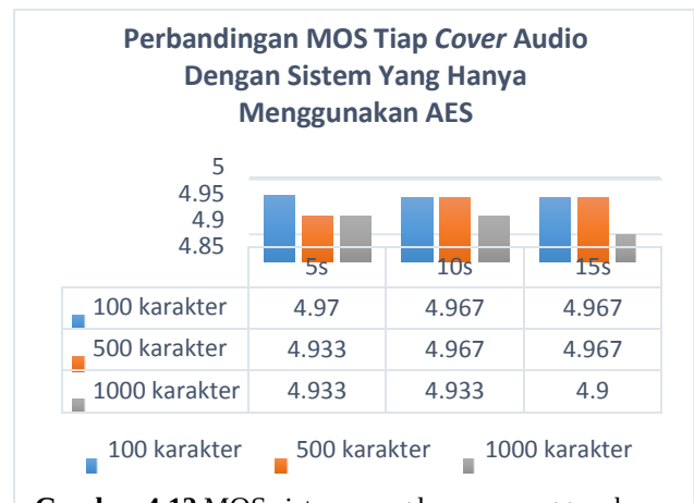
Gambar 4.12 MOS sistem yang hanya menggunakan AES tanpa pemodelan psychoacoustic
