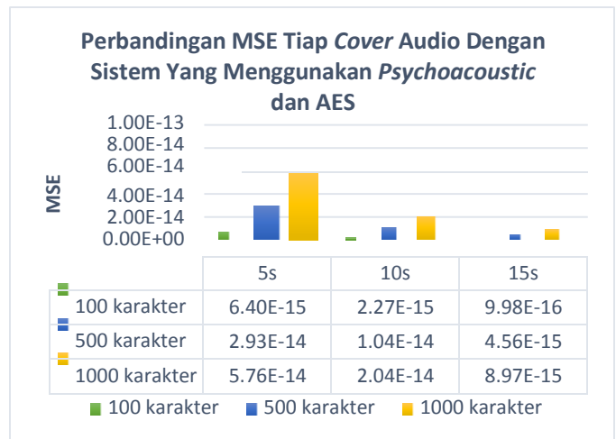
Gambar 4.2 MSE pengujian sistem yang menggunakan psychoacoustic dan AES
