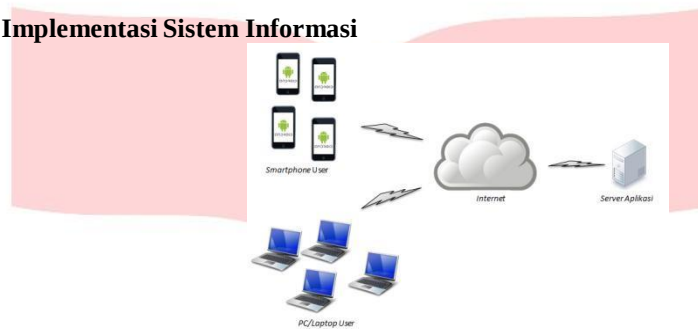
Gambar 2.2 Skema Implementasi
