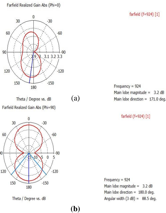
Gambar 4 Pola Radiasi Hasil Simulasi (a) Azimuth (b) Elevasi
