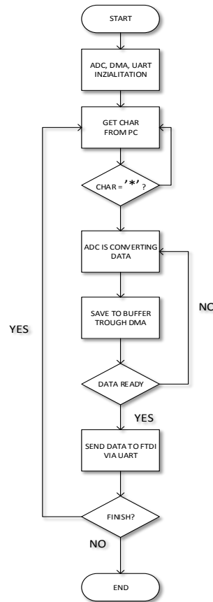
Gambar 1. Flowchart Perangkat Lunak Mikrokontroler
