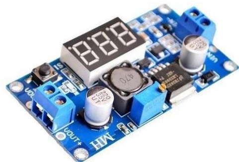
GAMBAR 10 MODUL LM2596
