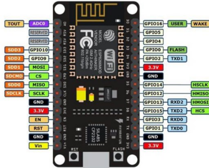
GAMBAR 2 ESP 8266
