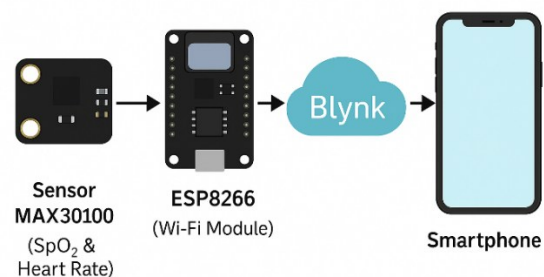
GAMBAR 6 DESAIN PERANCANGAN SISTEM DETEKSI DETAK JANTUNG DAN SATURASI OKSIGEN
