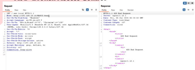
Gambar 11. Hasil request proxy menggunakan Burpsuite.
