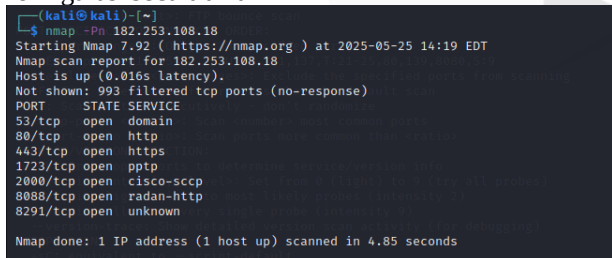
GAMBAR 2. Pemindaian menggunakan Nmap
