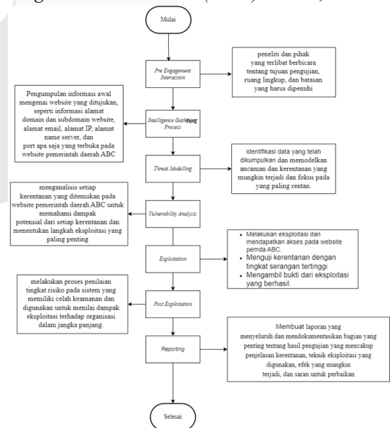
GAMBAR 2 Implementasi PTES
