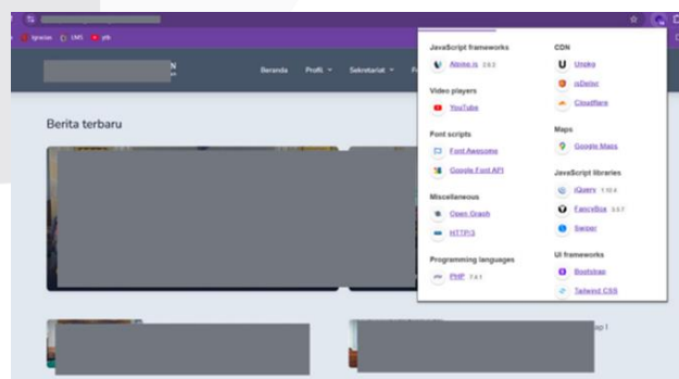
GAMBAR 5 Hasil Wappalyzer
