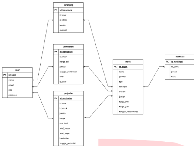
GAMBAR 6 ERD Sistem
