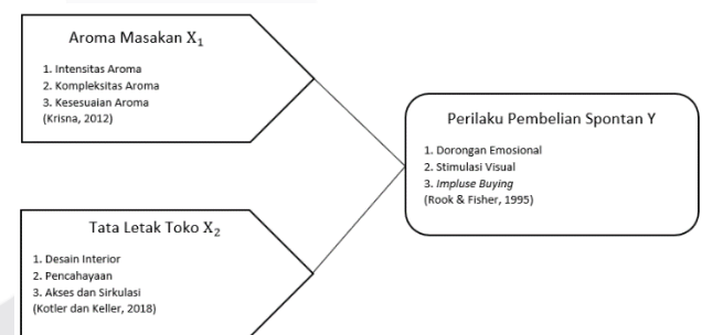
GAMBAR 2 Kerangka Pemikiran
