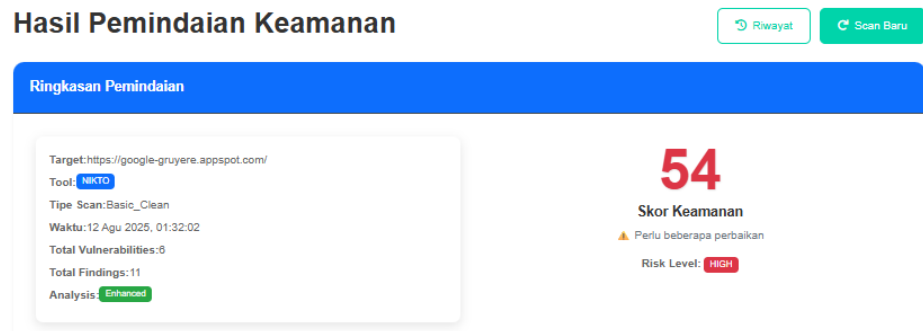
Gambar 5. 73 Skor Keamanan Website https://google-gruyere.appspot.com/ Berdasarkan Hasil Pemindaian Nikto
