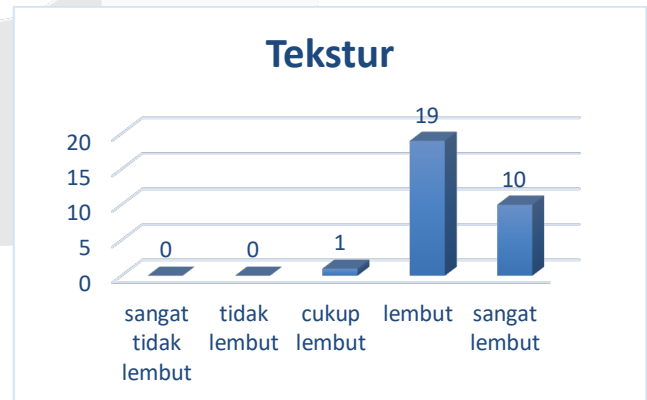
Gambar 5 Atribut Tekstur
