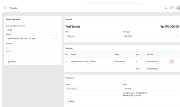
GAMBAR 8 (Halaman Transaksi)
