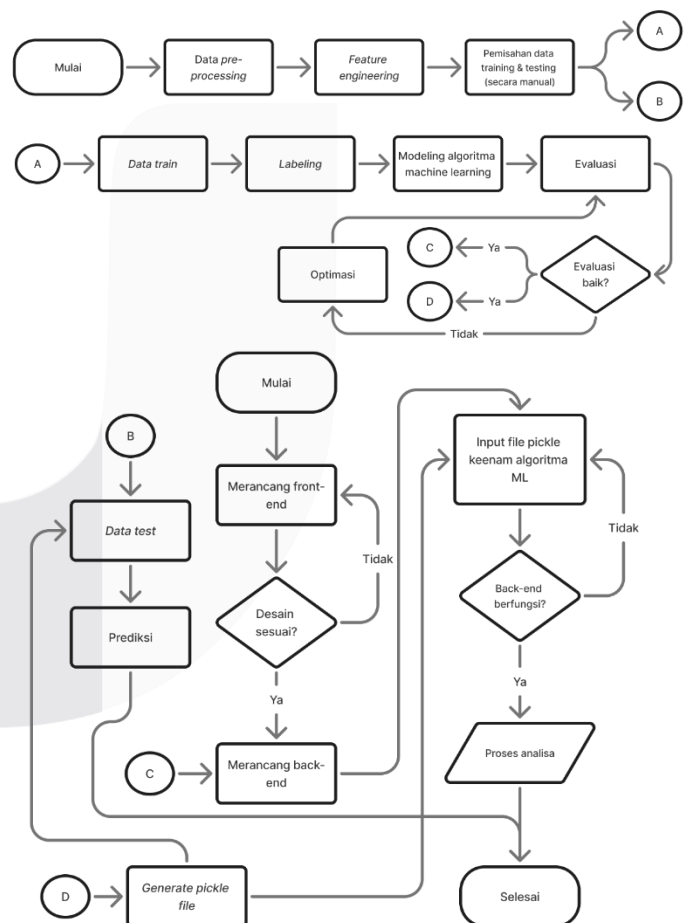
Gambar 4. Sistem Usulan
