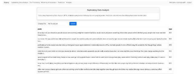
Gambar 9. Tahap EDA
