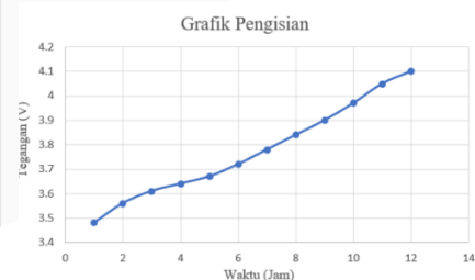
Gambar 5. Grafik pengisian daya pada baterai IoT.
