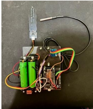
Gambar 4. Keseluruhan perangkat IoT.
