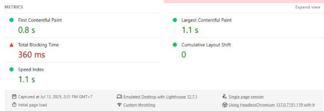
GAMBAR 6 HASIL PENGUJIAN SETIAP METRIKS PADA DESKTOP
