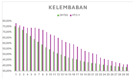
GAMBAR 8 GRAFIK PERBANDINGAN DETEKSI KELEMBABAN ANTARA DHT22 DAN THERMOMETER HTC-1
