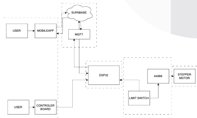
Gambar 3.3 Blok diagram sistem
