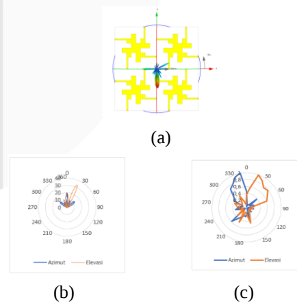
Gambar 11 Grafik Perbandingan Pola Radiasi Switchbeam Microstrip Antenna 4 Elemen Port 1 (a) Simulasi 3D; (b) Simulasi Polar; (c) Pengujian.
