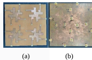
Gambar 10 Hasil Fabrikasi Switchbeam Antenna 4 Elemen (a) Tampak Depan; (b) Tampak Belakang
