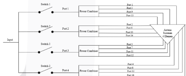
Gambar 4 (Blok Sistem Switchbeam Microstrip Antenna Susunan 4 Elemen)
