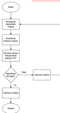
Gambar 1 (Flowchart Pembuatan Antena)
