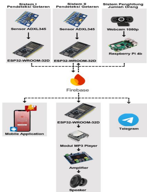
Gambar 1 Diagram Rangkaian
