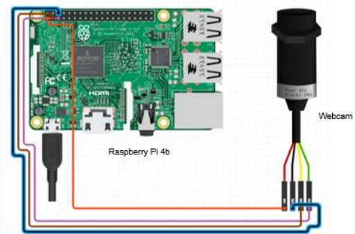
Gambar 4. Skematik Sub Sistem Penghitung Jumlah Orang
