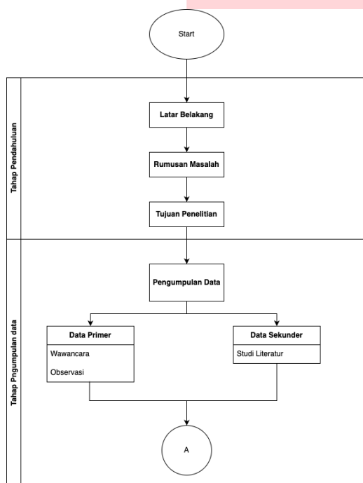
Gambar 2 Sistematika perancangan
