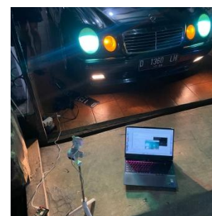
GAMBAR 3 (Setup Pengujian Sistem)
