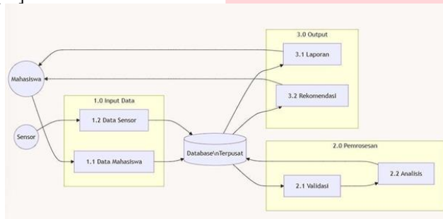
Gambar 1 (Arsitektur diagram)
