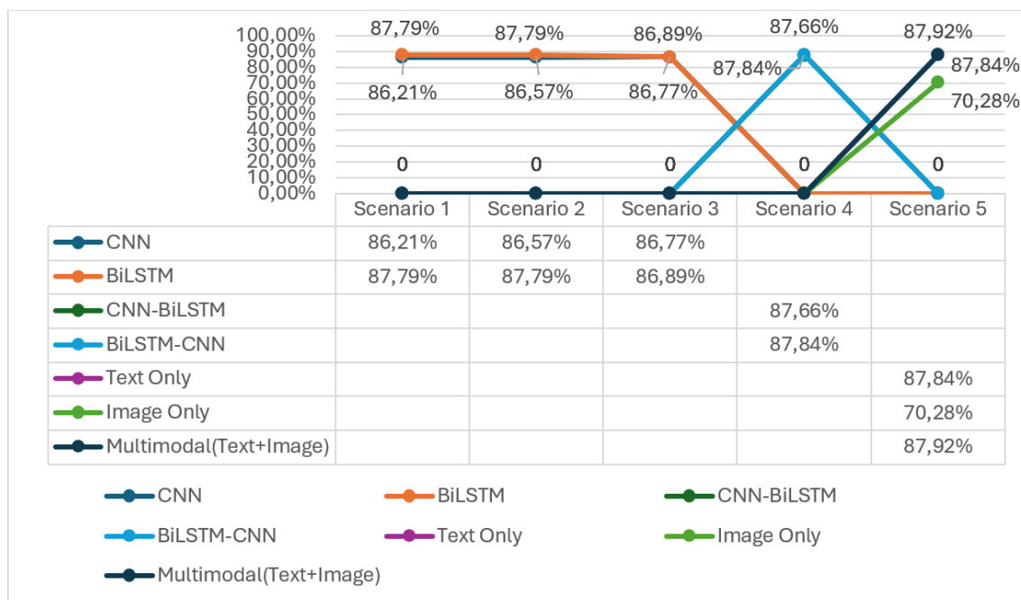
Gambar 6. Performa Akurasi Varian Model pada seluruh skenario
