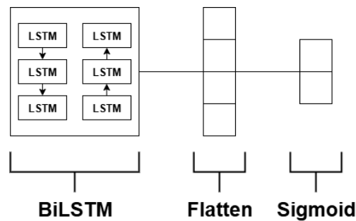
Gambar 3. Arsitektur BiLSTM
