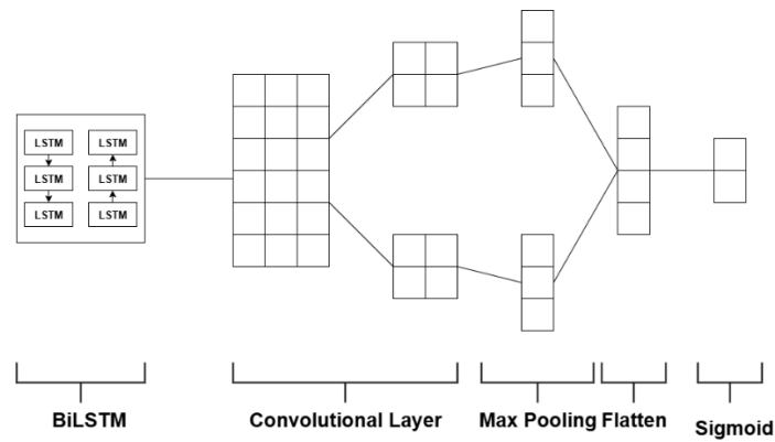
Gambar 5. Arsitektur BiLSTM-CNN
