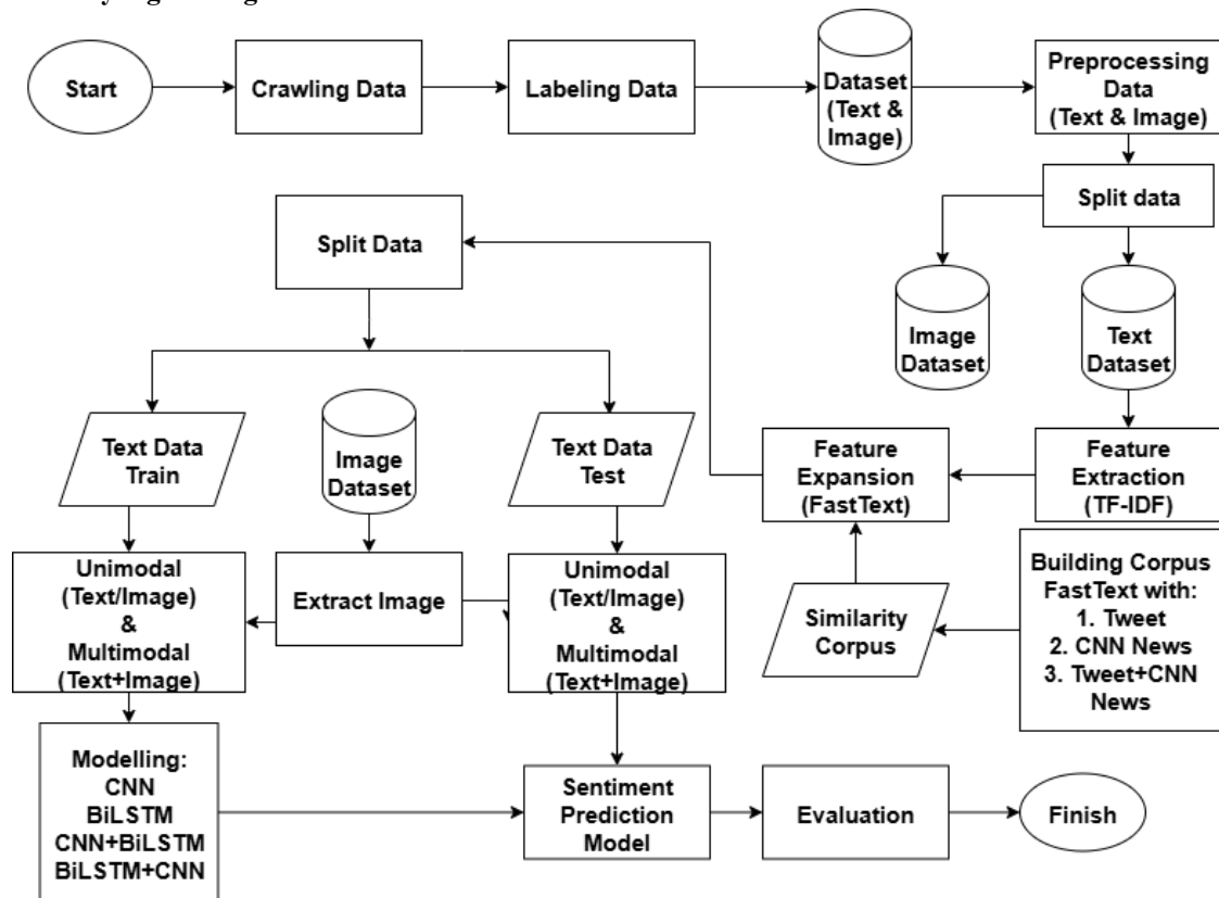
Gambar 1. Alur kerja sistem menggunakan arsitektur hibrida CNN-BiLSTM
