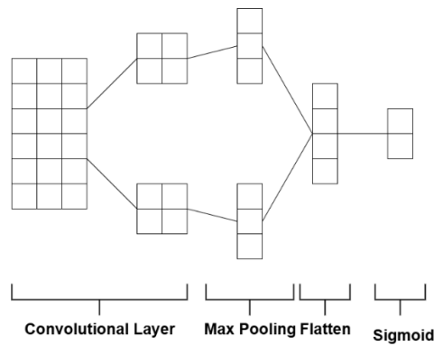
Gambar 2. Arsitektur CNN[16]
