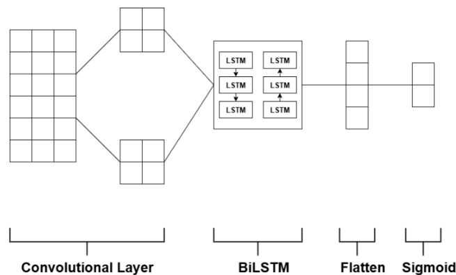
Gambar 4. Arsitektur CNN-BiLSTM
