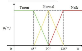
Gambar III. 3 Fuzzifikasi motor servo
