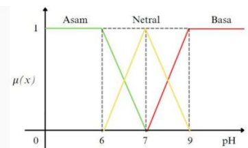
Gambar III. 2 Fuzzifikasi pH air
