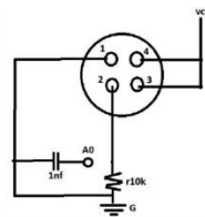
Gambar II. 3 Rangkaian modul sensor TGS2602
