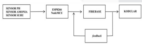
Gambar III. 6 Desain Sistem Komunikasi IoT
