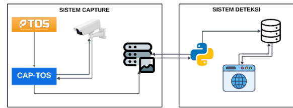
Gambar 2 Desain sistem
