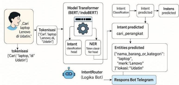
Gambar 4 Perancangan Chatbot Intent & NER
