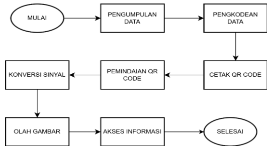
Gambar 2 Pengembangan QR Code
