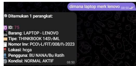
Gambar 14 Pencarian Perangkat
