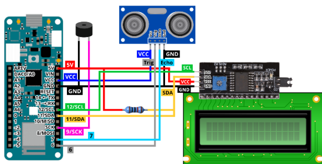
GAMBAR 2 Rancangan Alat
