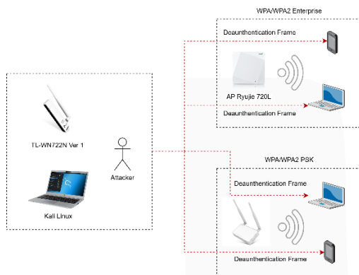
Gambar 8 Simulasi Serangan dengan Deauthentication
