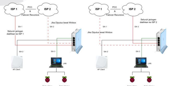
Gambar 6 Skenario Kedua Pengujian Failover Jaringan
