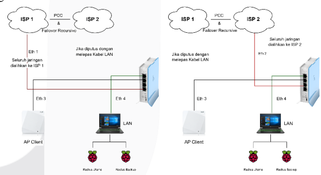
Gambar 5 Skenario Pertama Pengujian Failover Jaringan
