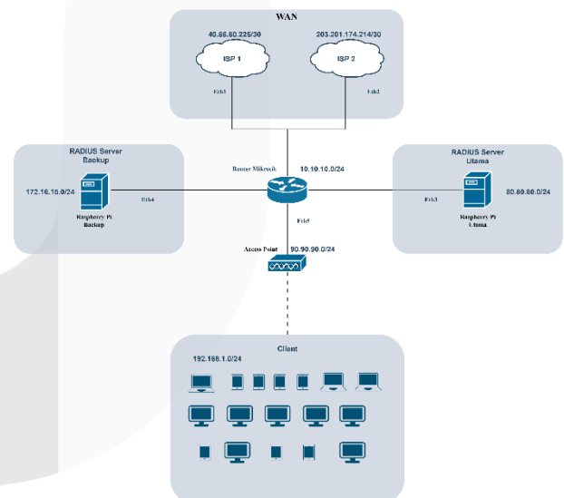
Gambar 1 Topologi Jaringan
