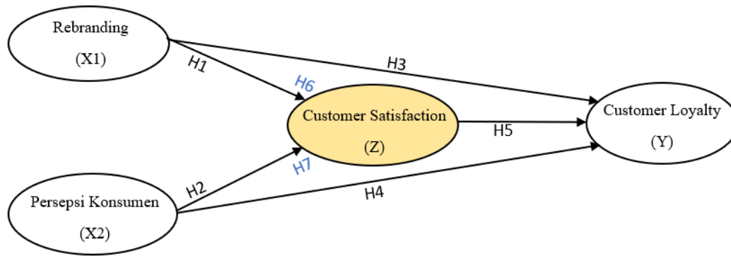
Gambar 2.1 Kerangka Pemikiran
