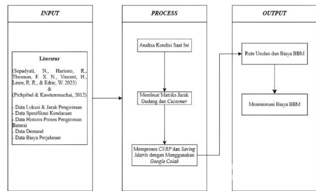
GAMBAR 5 Kerangka Berpikir
