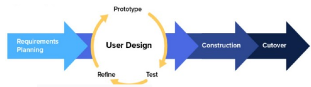
GAMBAR 1 (METODE RAD)
