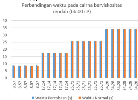
Gambar 6 Perbandingan waktu percobaan dan waktu normal pada viskositas rendah
