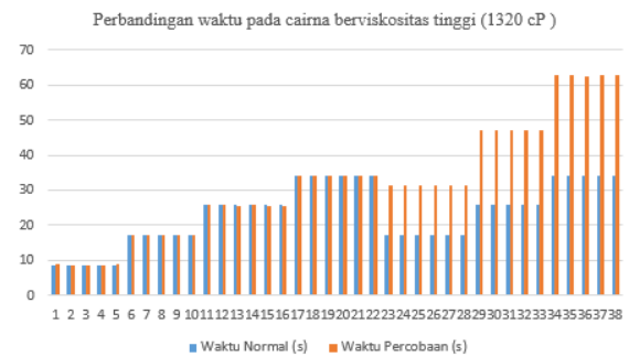
Gambar 7 Perbandingan waktu percobaan dan waktu normal pada viskositas tinggi
