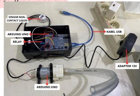
Gambar 4 Rangkaian Alat
