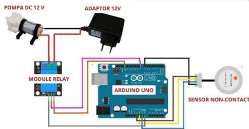
Gambar 3 Diagram Skema Perangkat
