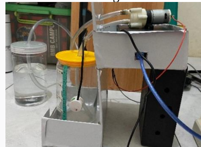
Gambar 5 Perangkat Prototipe
