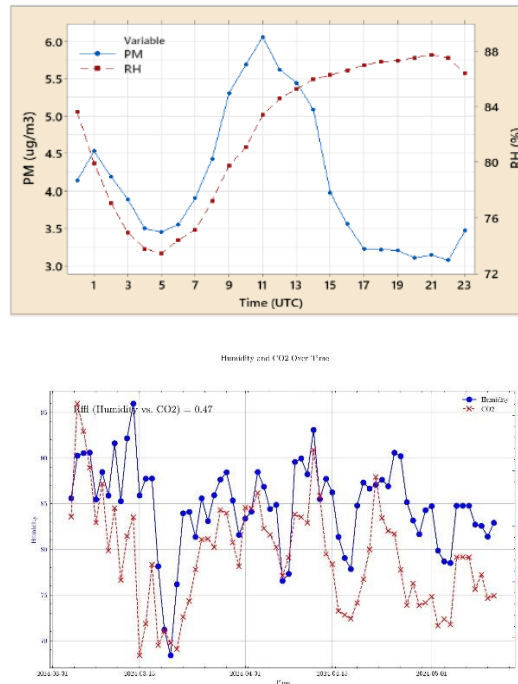
Gambar 1. 1 Grafik Perbandingan Kelembapan, \text{PM}_{2.5} , dan \text{CO}_2
