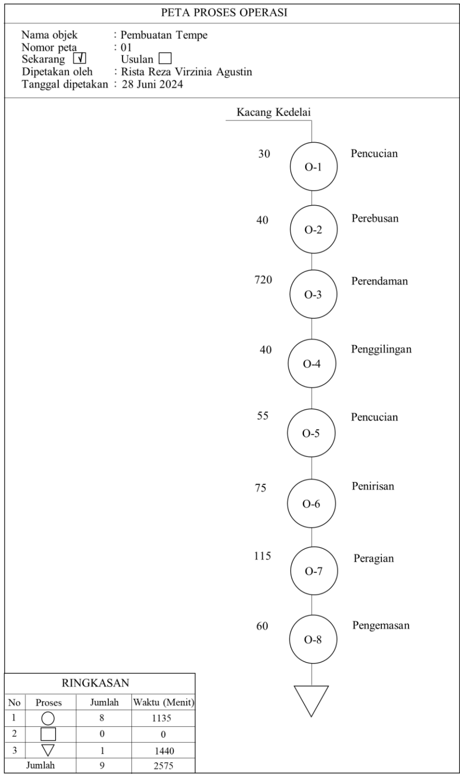
Gambar I. 7. Peta Proses Operasi
