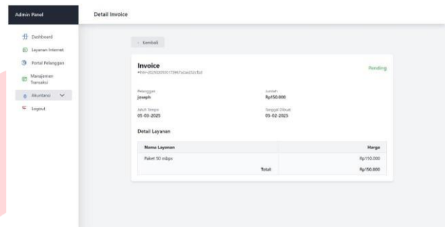
GAMBAR 4 (Detail Transaksi)
