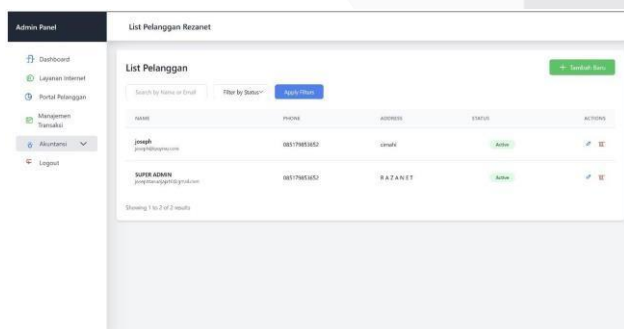
GAMBAR 2 (List Pelanggan)
