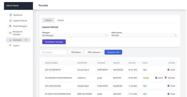
GAMBAR 3 (Transaksi
