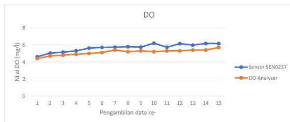
Gambar 19. Hasil pengukuran DO dengan menggunakan aerator.
