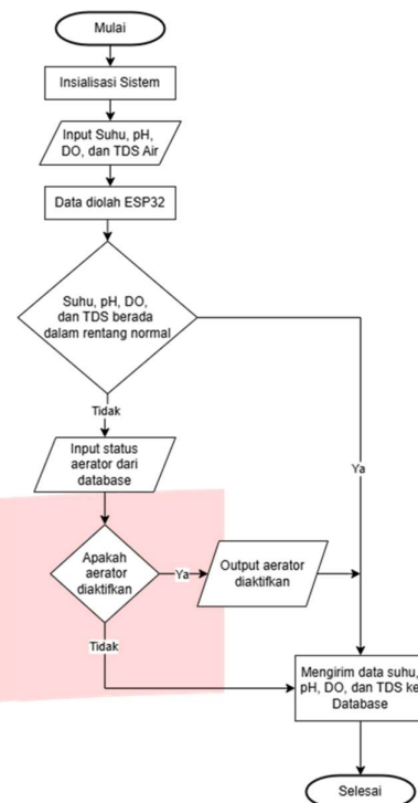
Gambar 3. Flowchart Perangkat IoT
