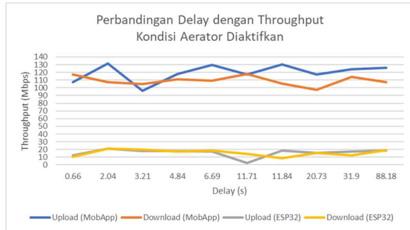
Gambar 26. Hasil SpeedTest ketika Aerator diaktifkan
