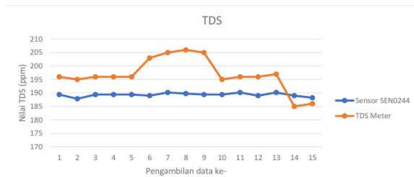
Gambar 21. Hasil pengukuran TDS menggunakan aerator.
