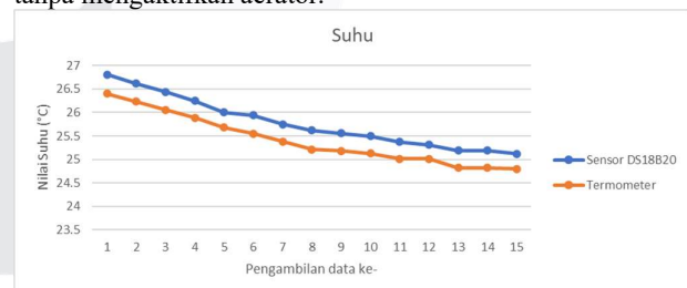
Gambar 14. Hasil Pengukuran Suhu tanpa Aerator
