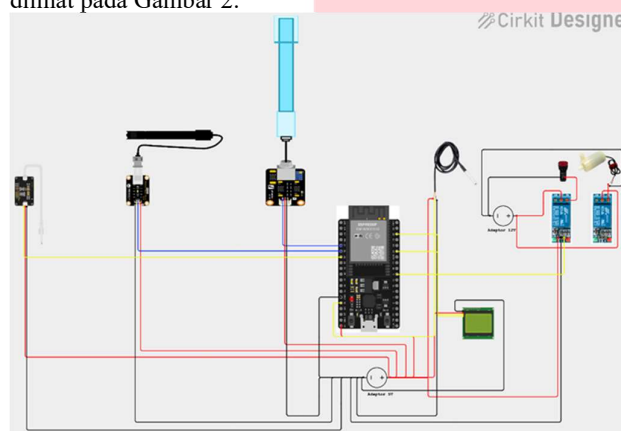
Gambar 2. Wiring Perangkat IoT
