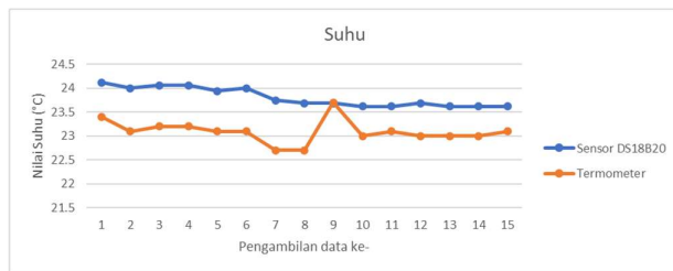
Gambar 15. Hasil Pengukuran Suhu dengan Aerator
