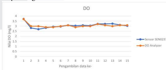
Gambar 18. Hasil pengukuran DO tanpa menggunakan aerator.
