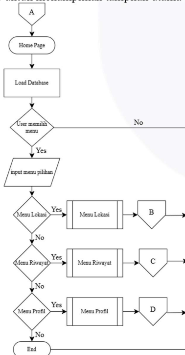
Gambar 5. Flowchart Halaman Utama
