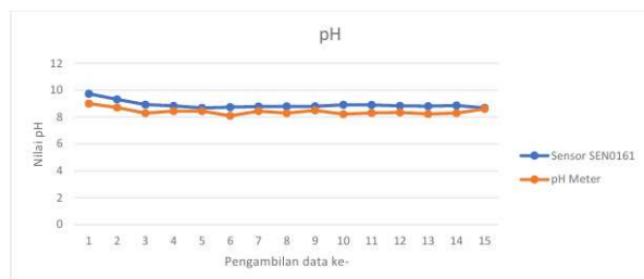
Gambar 17. Hasil pengukuran pH dengan menggunakan aerator.
