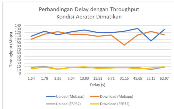
Gambar 25. Hasil SpeedTest ketika Aerator dimatikan
