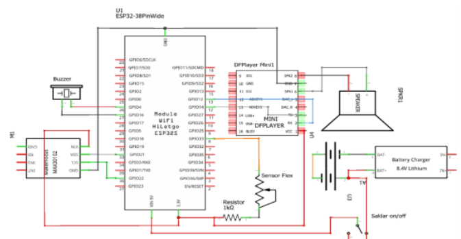
GAMBAR 3.4 SKEMATIK RANGKAIAN
