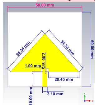
Gambar 3. Geometri Dimensi Patch tunggal Triangular.
