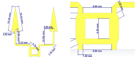
Gambar 5. Dimensi Antena Butler Matrix 2x2 Dengan Lapisan superstrat Menggunakan FR-4.
