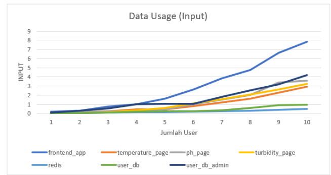
GAMBAR 16 (Data Usage(Input))
