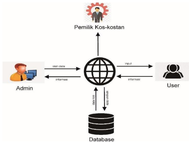
GAMBAR 3 (Arsitektur Sistem)
