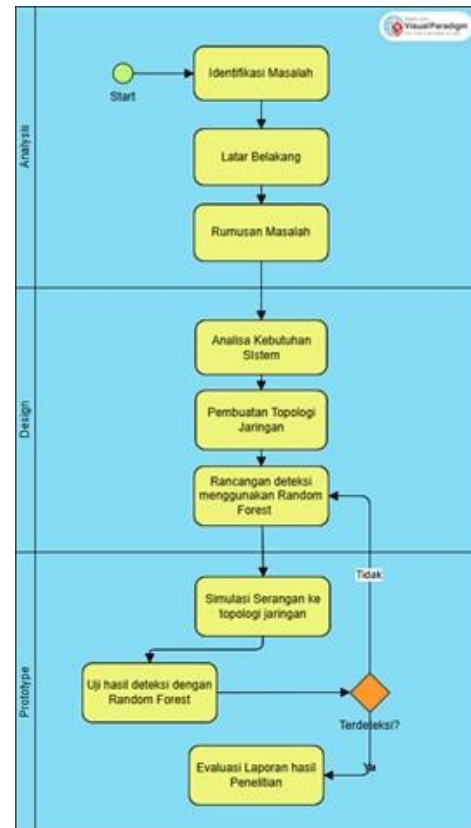
Gambar III.2 Sistematika Penyelesaian Masalah
