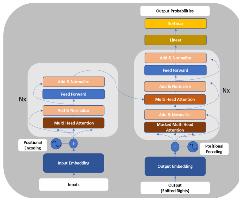
Gambar 1. Arsitektur Transformer
