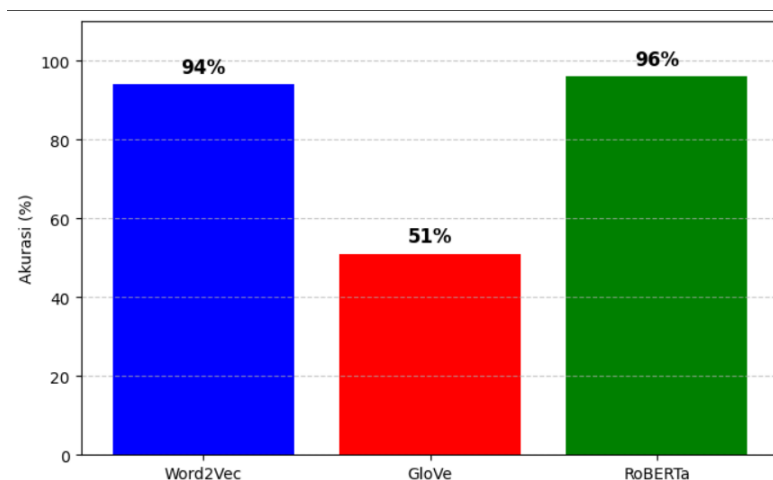
Gambar 6. Perbandingan Akurasi
