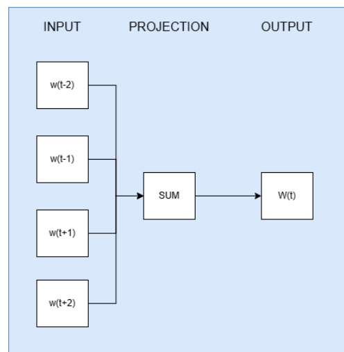
Gambar 2. Tahapan CBOW
