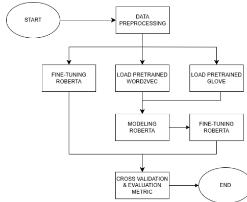
Gambar 4. Rancangan Sistem
