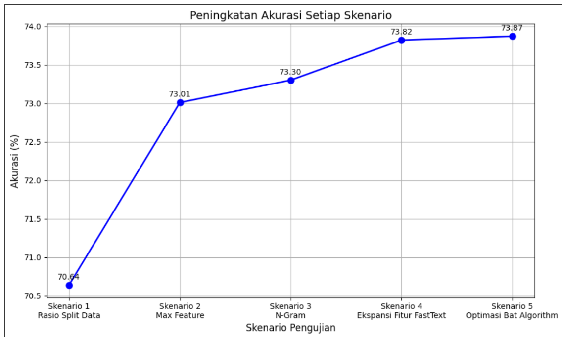
Gambar 6. Fluktuasi Setiap Skenario
