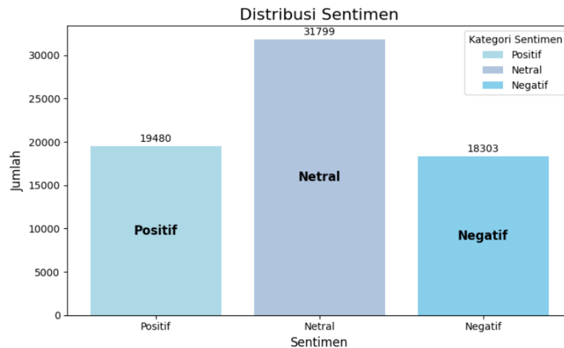
Gambar 2 Distribusi Sentimen setelah Preprocessing
