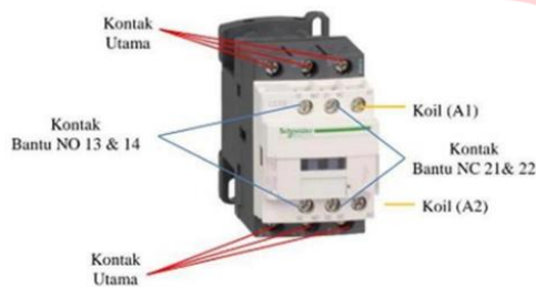
GAMBAR 5 (KONTAKTOR [8])
