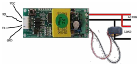
GAMBAR 4 (PZEM-004T [7])
