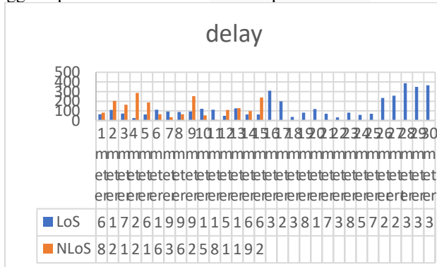
GAMBAR 26 (GRAFIK PERBANDINGAN DELAY LOS DAN NLOS)
