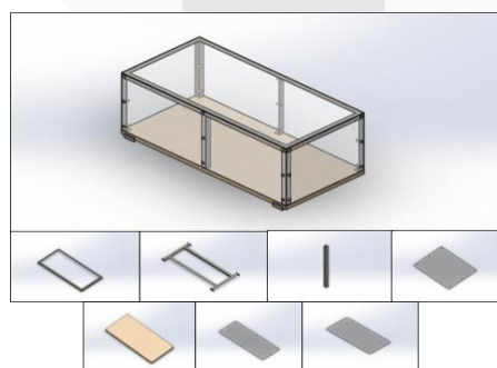
Gambar 1 Assembly peti Sumber: dokumentasi penulis, 2024
