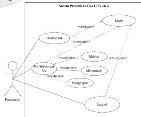
Gambar 7 (Usecase Diagram Pangkalan)
