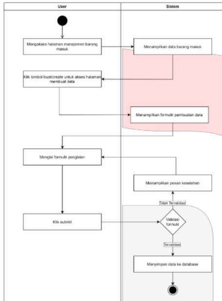
Gambar 8 (Activity Diagram Menambahkan Barang Masuk)
