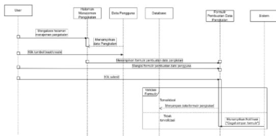
Gambar 9 (Sequence Diagram Menambahkan Data Pangkalan)
